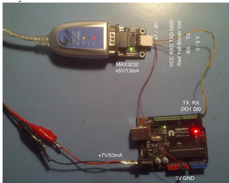
Рисунок 8. Вариант подключения контроллера Arduino UNO к преобразователю USB-COM компьютера.
