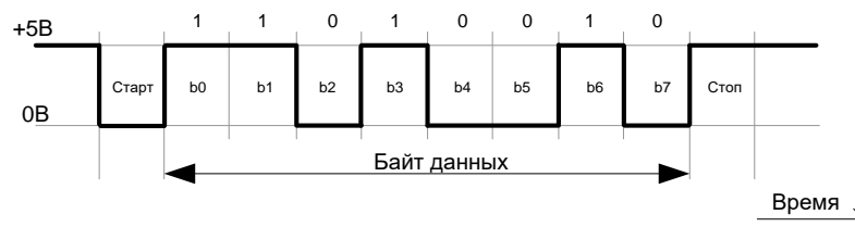
Рисунок 2. Временная диаграмма UART последовательной передачи данных (01001011 2 ) микросхемы ATmega328P контроллера Arduino UNO.
