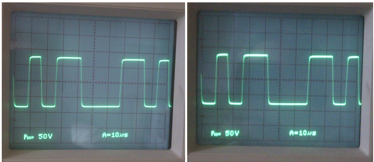
Рисунок 11. Сигнал амплитудой +7.5/-8 В на концах RS-232 линии составного кабеля длиной 9,5 м. Частота передачи данных 115200 бит/с. Сигнал не имеет заметных искажений.
