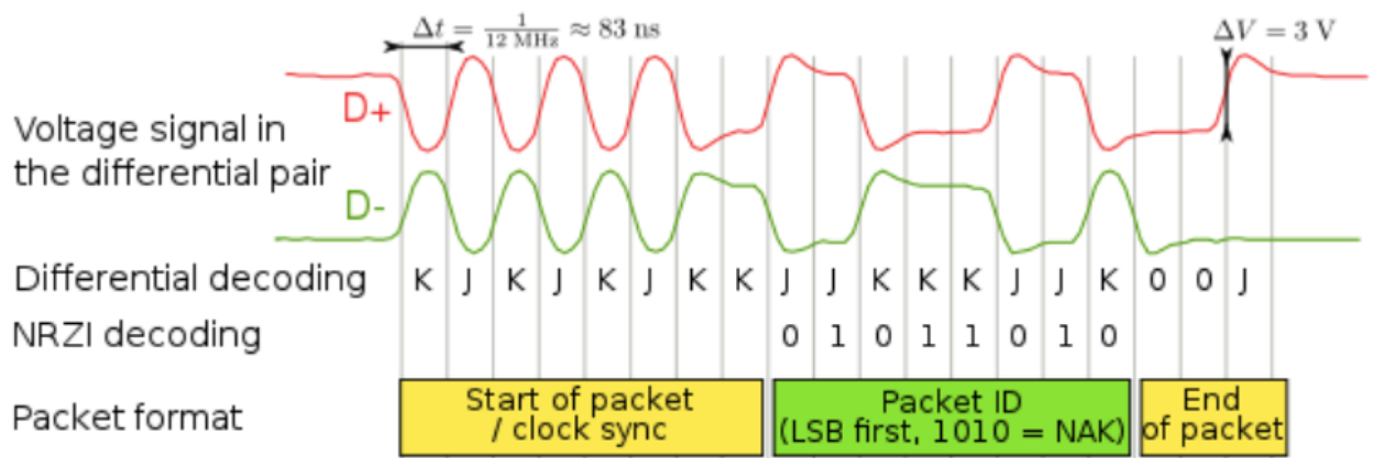
Рисунок 4. Пример передачи пакета по дифференциальной линии USB 1.1 в режиме Full-speed [2]. Изменение состояние дифференциального сигнала соответствует передаче нуля, сохранение уровней - соответствует передаче единицы. Для улучшения синхронизации на единичных последовательностях принудительно вставляют ноль на каждые 6 единиц подряд.
