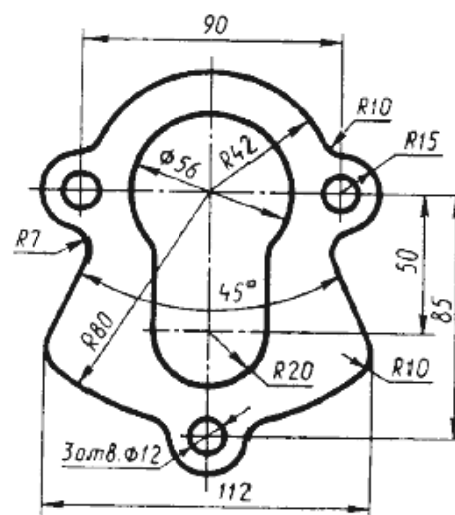
Чертеж 20
