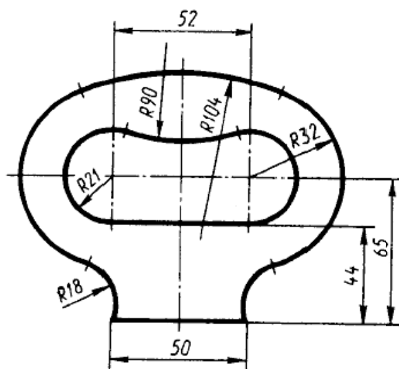
Чертеж 30
