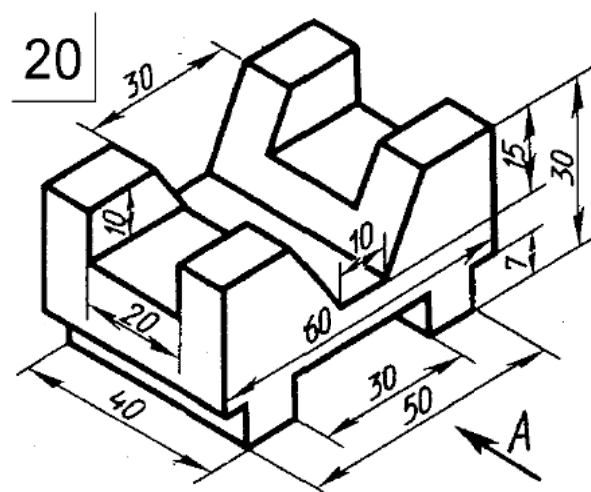
Чертёж 20
