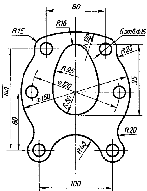
Чертёж 17
