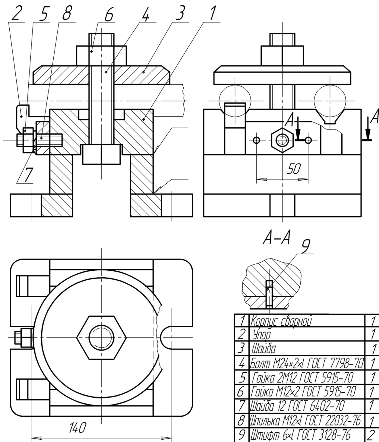
Чертёж 31 – Зажим
