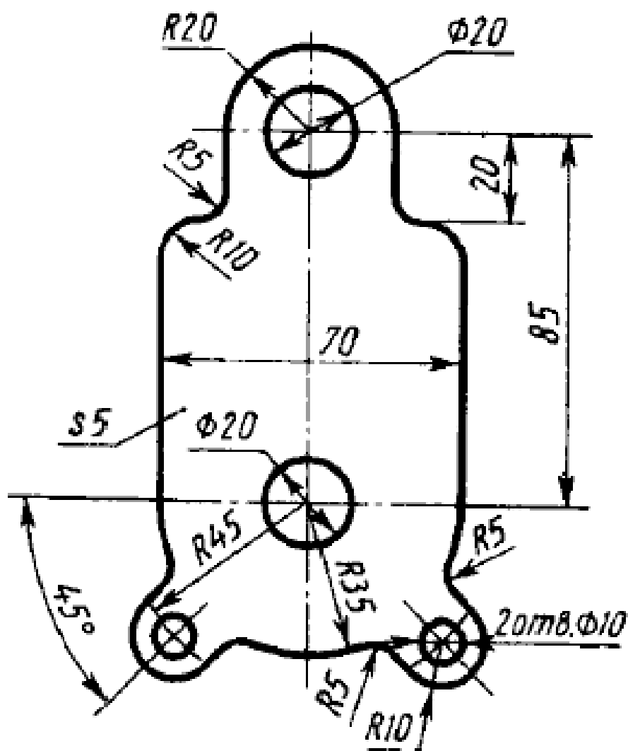
Чертеж 32
