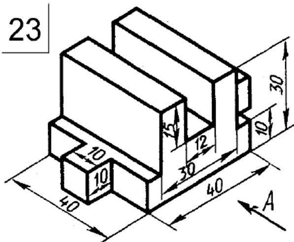
Чертёж 23
