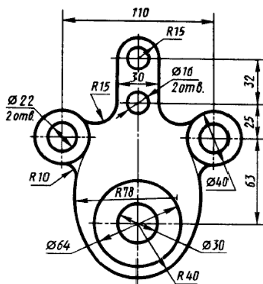
Чертеж 24
