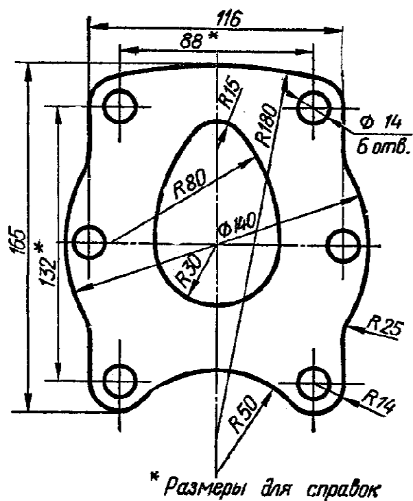
Чертеж 7
