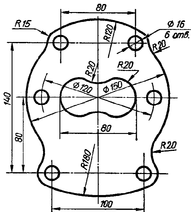
Чертеж 12
