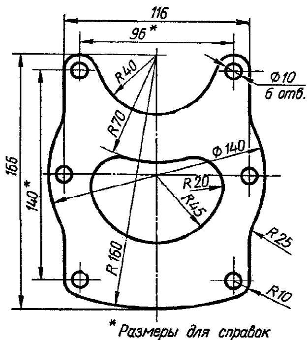
Чертеж 9
