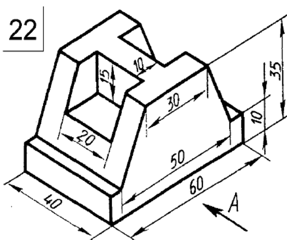
Чертёж 22
