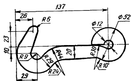
Чертеж 28
