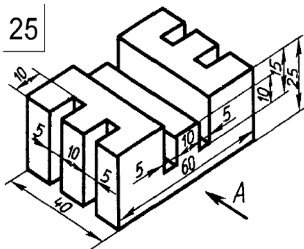
Чертёж 25
