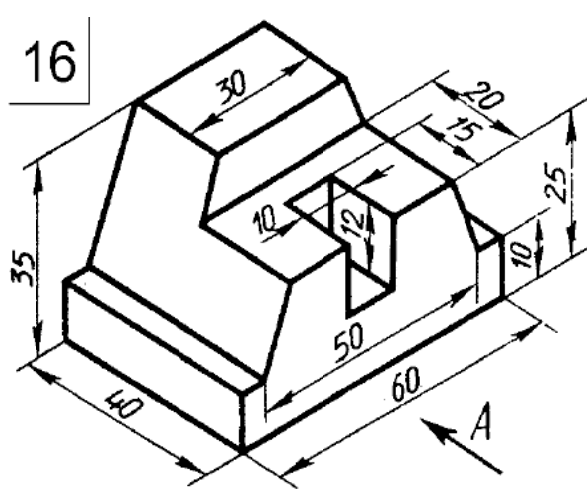
Чертёж 16
