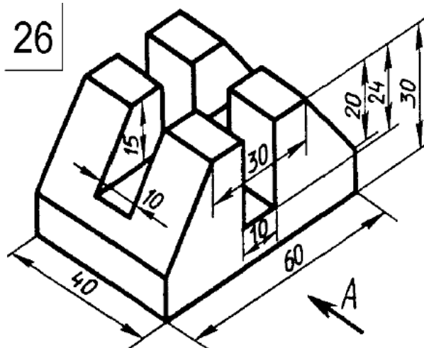
Чертёж 26
