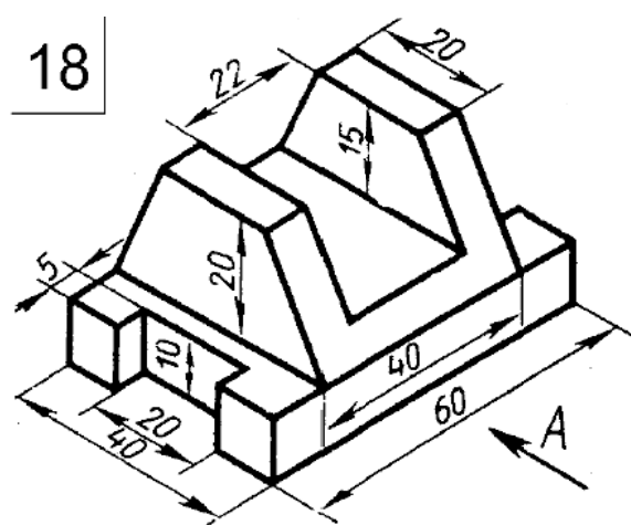
Чертёж 18
