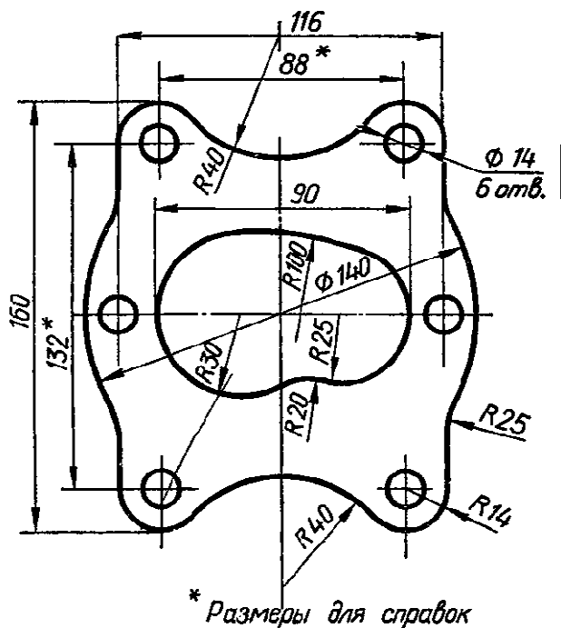
Чертёж 1
