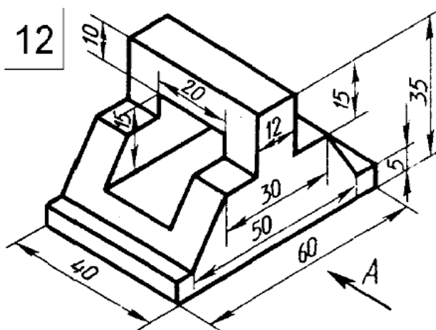
Чертёж 12
