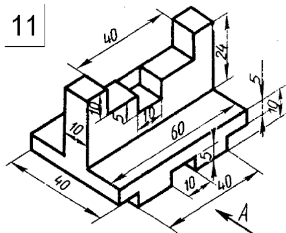
Чертёж 11
