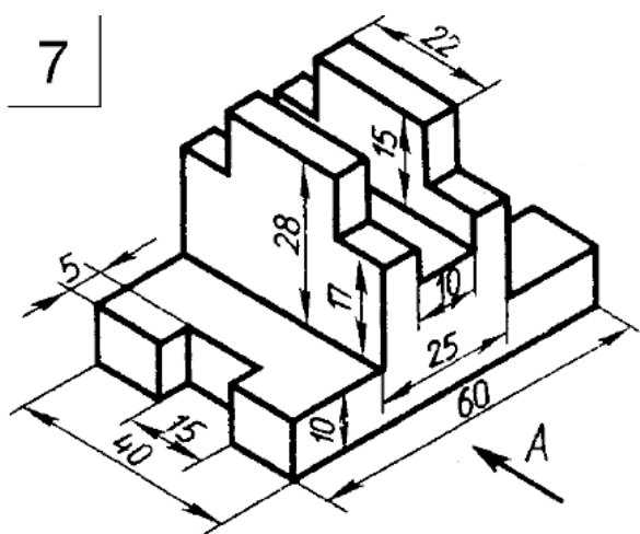
Чертёж 7
