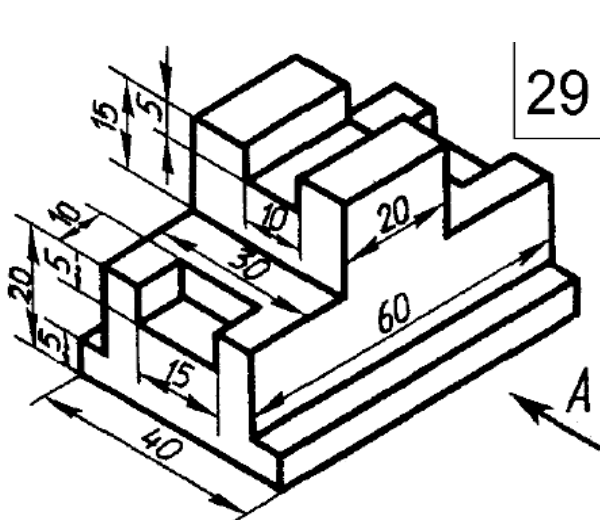
Чертеж 29
