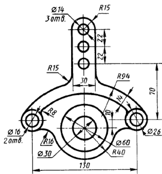
Чертеж 27
