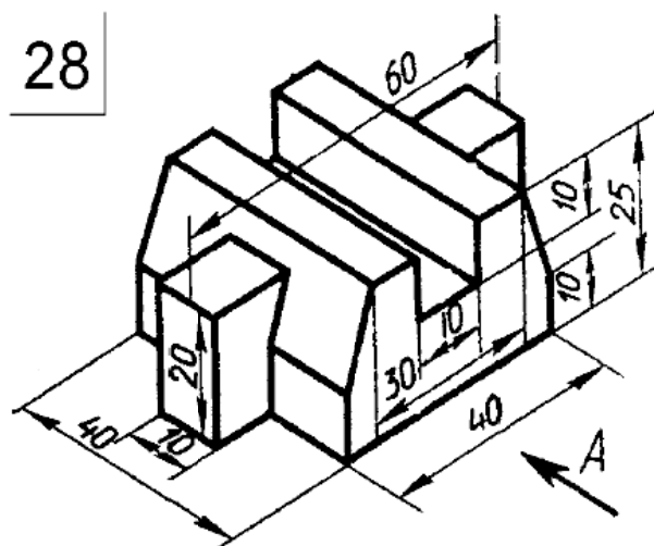
Чертёж 28
