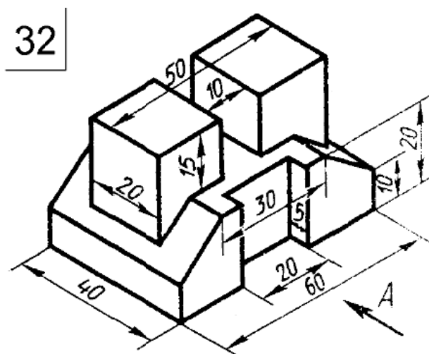
Чертеж 32
