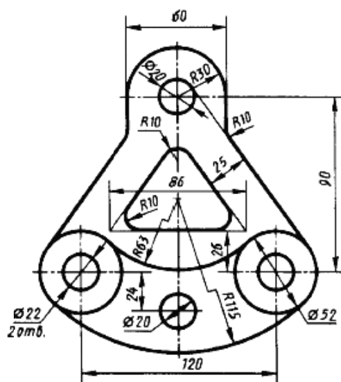
Чертеж 21
