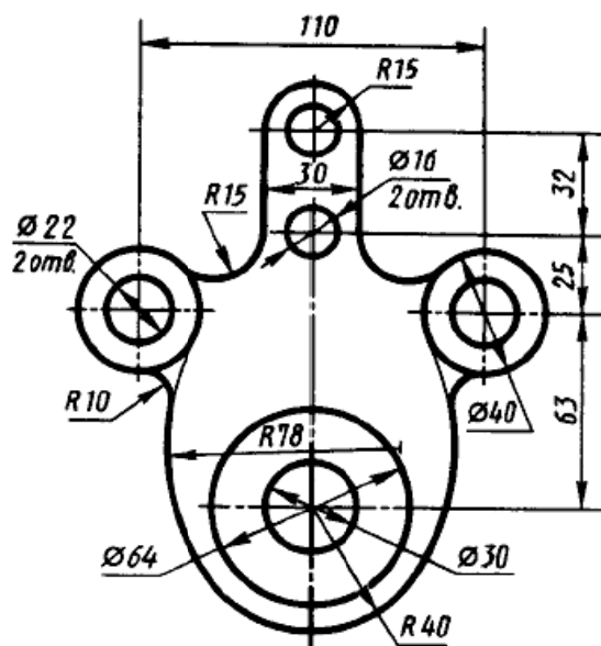
Чертеж 26
