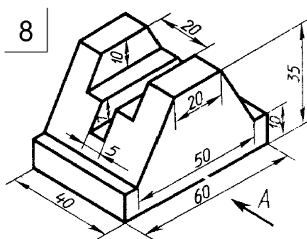
Чертёж 8
