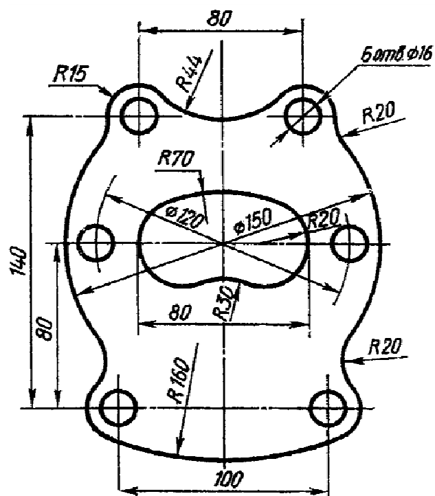
Чертёж 16
