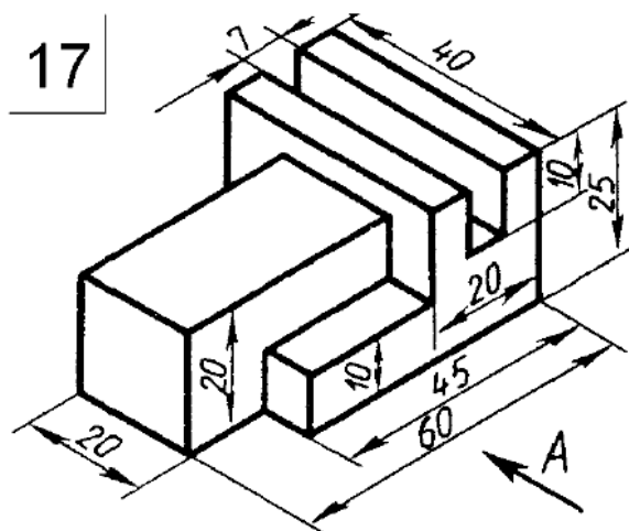
Чертёж 17
