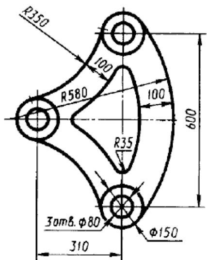
Чертеж 29
