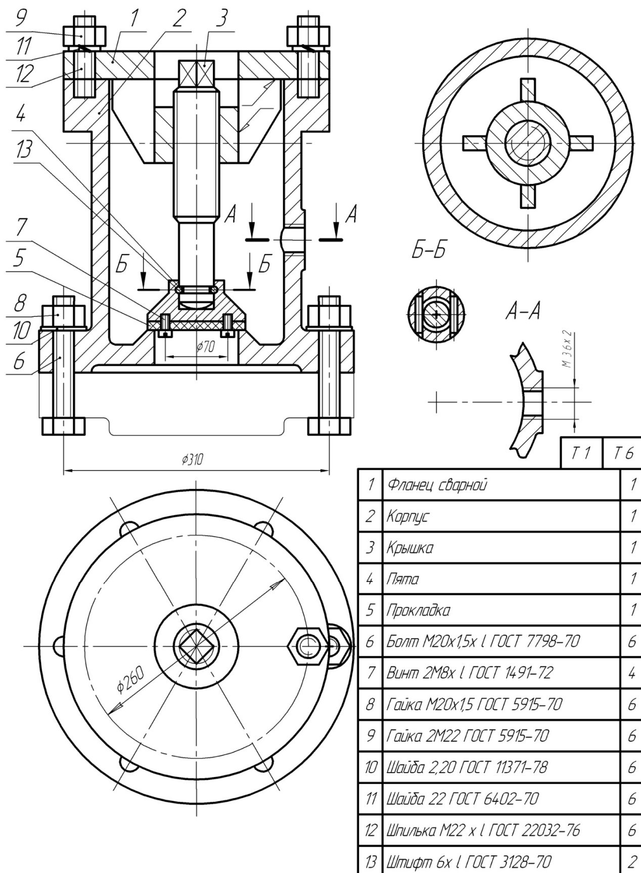
Чертёж 32 – Задвижка
