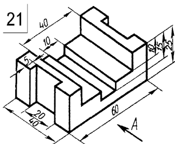
Чертёж 21
