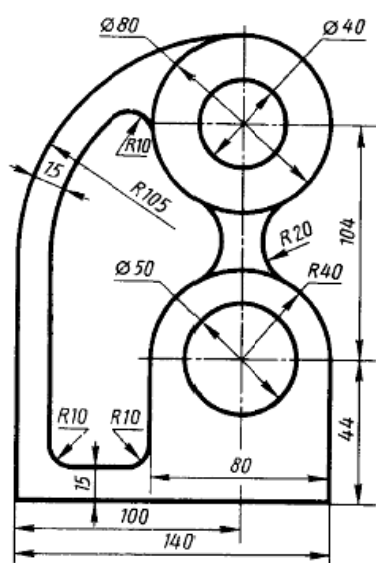
Чертеж 23
