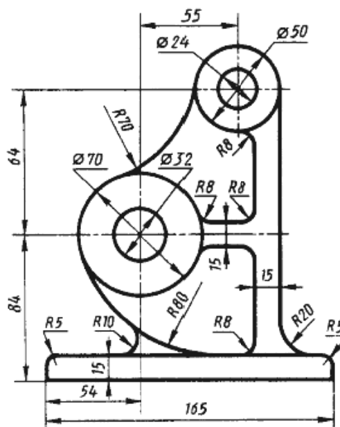
Чертеж 22
