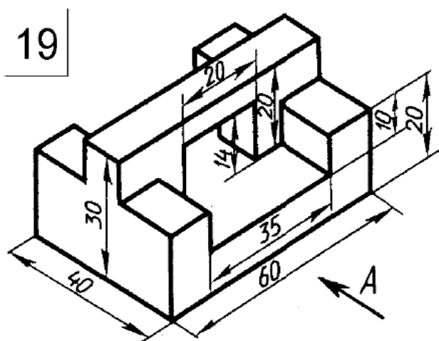
Чертёж 19
