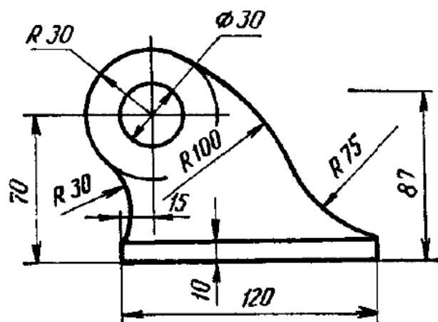
Чертеж 25
