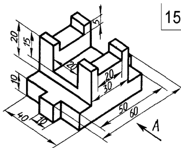
Чертёж 15
