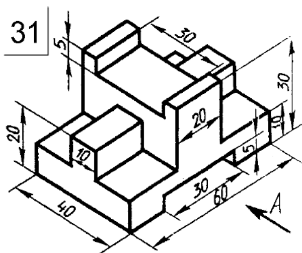
Чертеж 31
