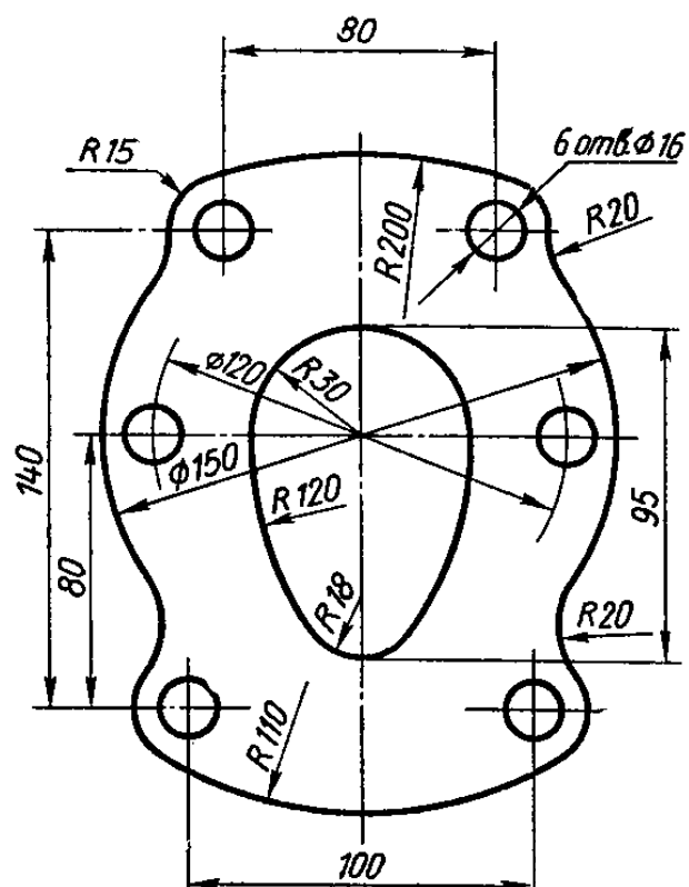
Чертёж 18
