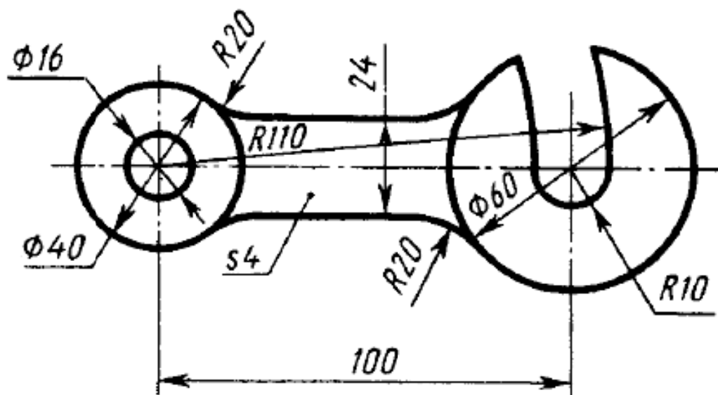
Чертеж 31
