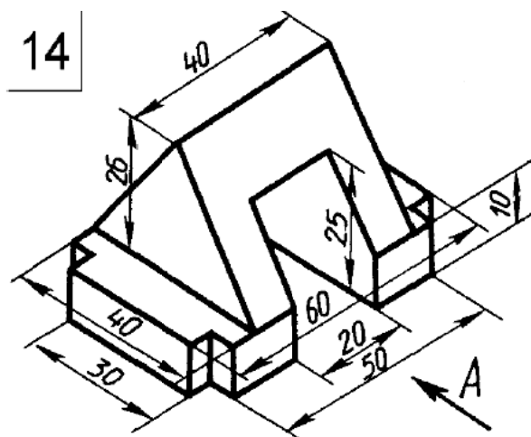
Чертёж 14
