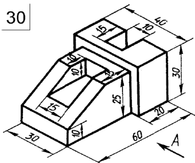
Чертеж 30
