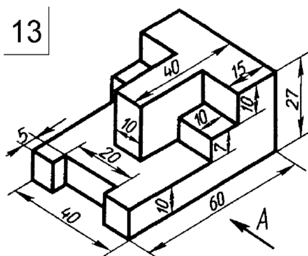
Чертёж 13
