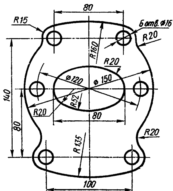
Чертеж 14
