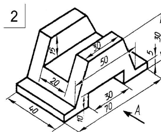
Чертёж 2
