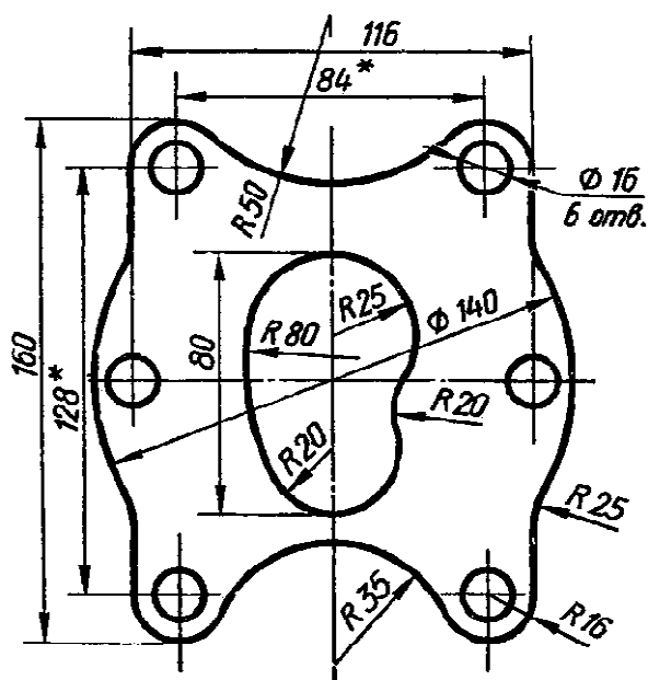
Чертёж 2
