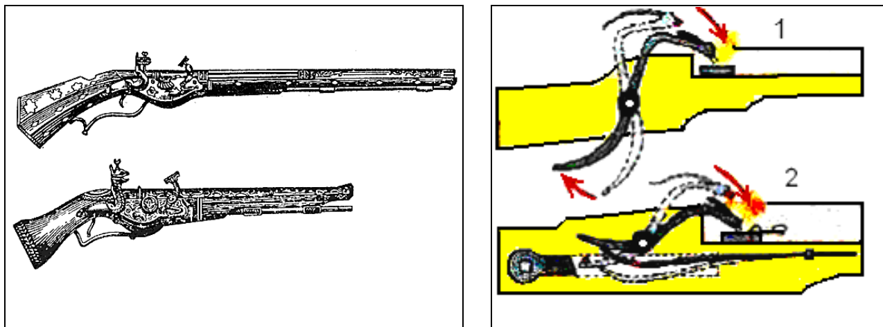
а – завесные пищали; б – варианты конструкции фитильного замка: 1 – серпентин; 2 – простейший замок с шепталом
