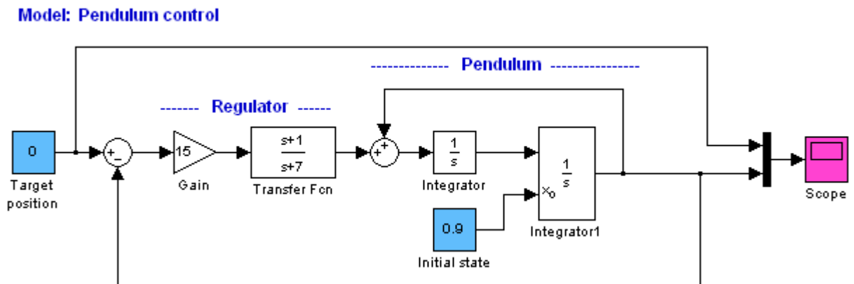
Рис. 3. Модель стабилизации маятника в верхнем положении.
