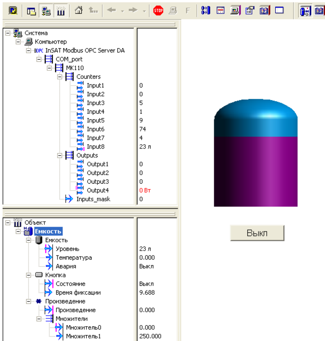
Рис. 3. Дерево объектов OPC сервера и SCADA клиента и мнемосхема частично заполненной цистерны с кнопкой включения ШИМ. Система находится в работе.
