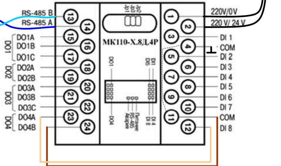
Рис. 1. Устройство дискретного ввода-вывода МК110-224.8Д.4Р. Схема подключения для выполнения лабораторной работы.
