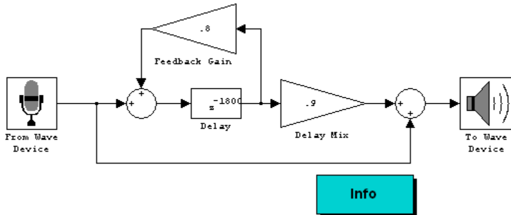
Рис. 13. Пример построения эффекта реверберации.
