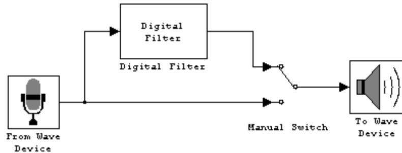
Рис. 11. Модель simulink.
